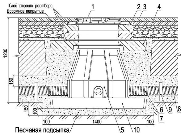
Рисунок Г.7 – Схема установки кабельного колодца ККТ-1-ССД
